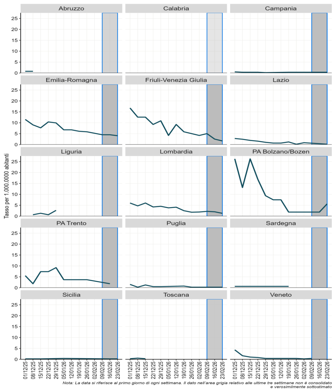
Figura 20 - Tasso di ospedalizzazione (per 1.000.000 ab.) per Regione/PPAA a partire dall'1 dicembre 2025
