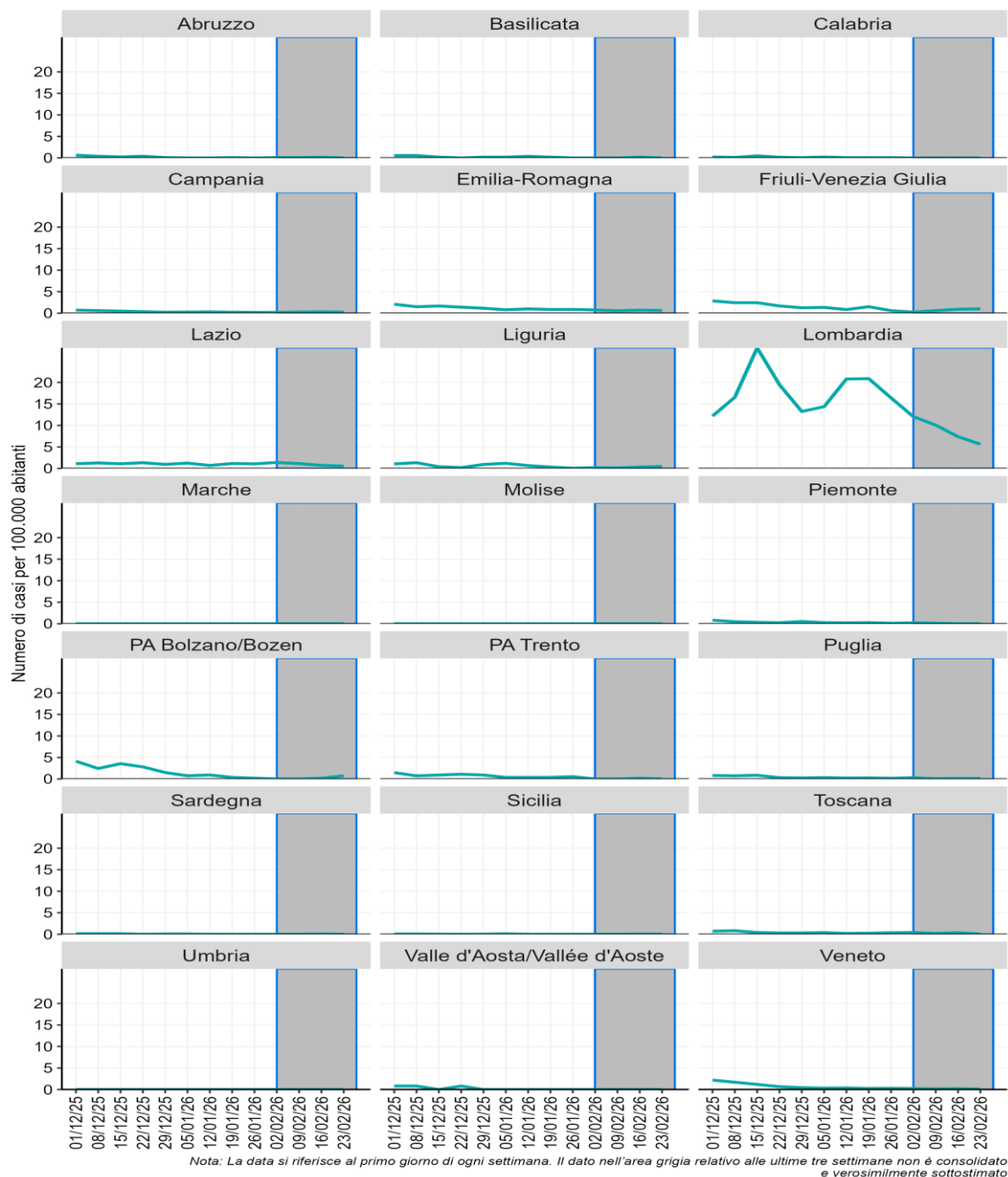
Figura 18 - Incidenza settimanale di diagnosi di infezioni per SARS-CoV-2 (per 100.000 ab.) per Regione/PPAA dall'1 dicembre 2025
