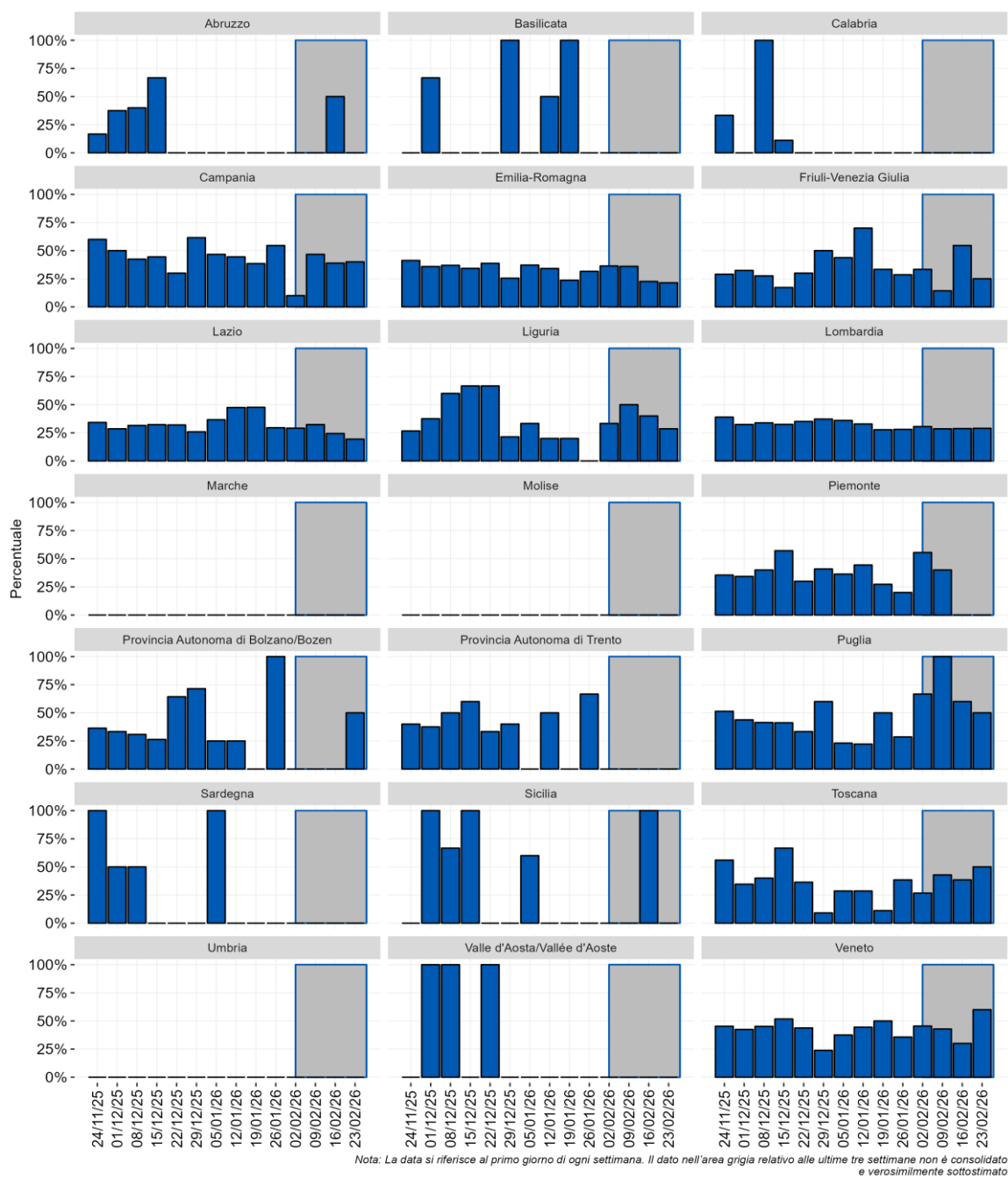
Figura 19 - Percentuale di reinfezioni per Regione/PPAA dall'1 dicembre 2025
