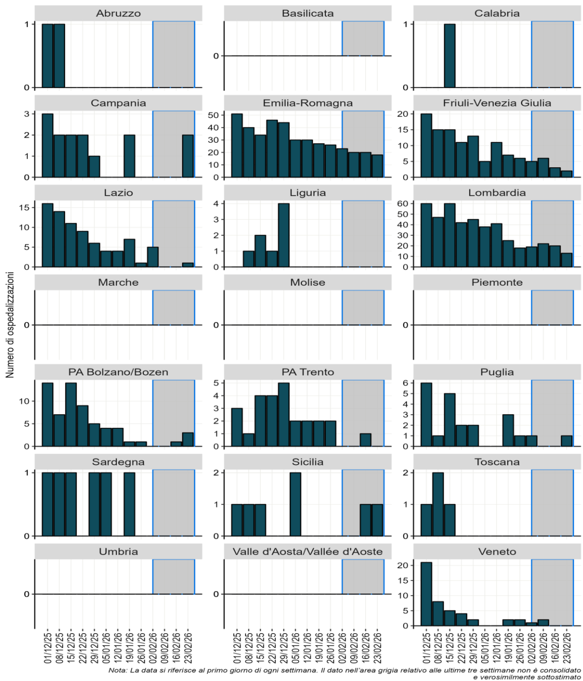
Figura 22 - Ricoveri settimanali in AM per Regione/PPAA dall'1 dicembre 2025
