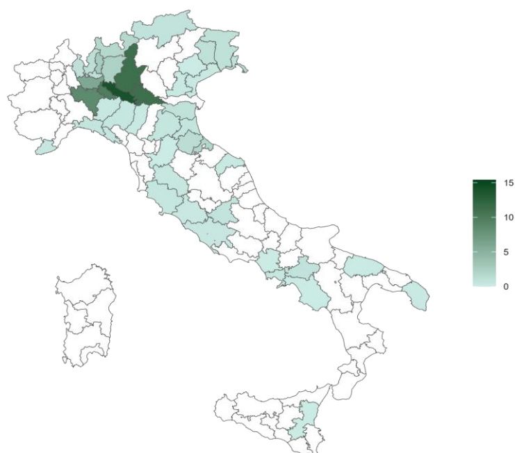
Figura 5 - Tasso di incidenza di infezioni da SARS-CoV-2 (per 100.000 ab.) segnalate in Italia per Regione/PA di domicilio/residenza (Periodo: 23/02 - 01/03/2026)
