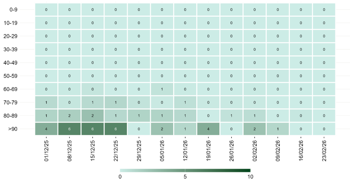
Figura 15 - Tasso settimanale di mortalità (per 1.000.000 ab.) per fascia d'età a partire dall'1 dicembre 2025
