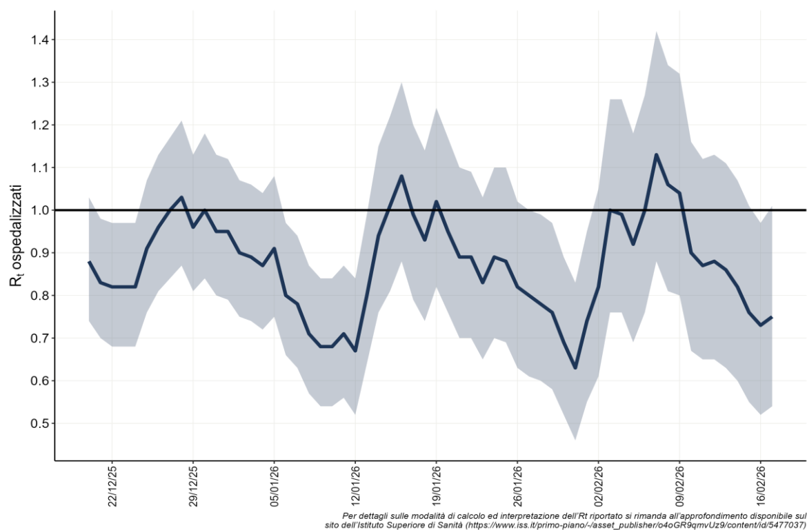
Figura 8 - Andamento giornaliero di Rt ospedalizzazioni nazionale, calcolato con dati estratti il 25 febbraio 2026
