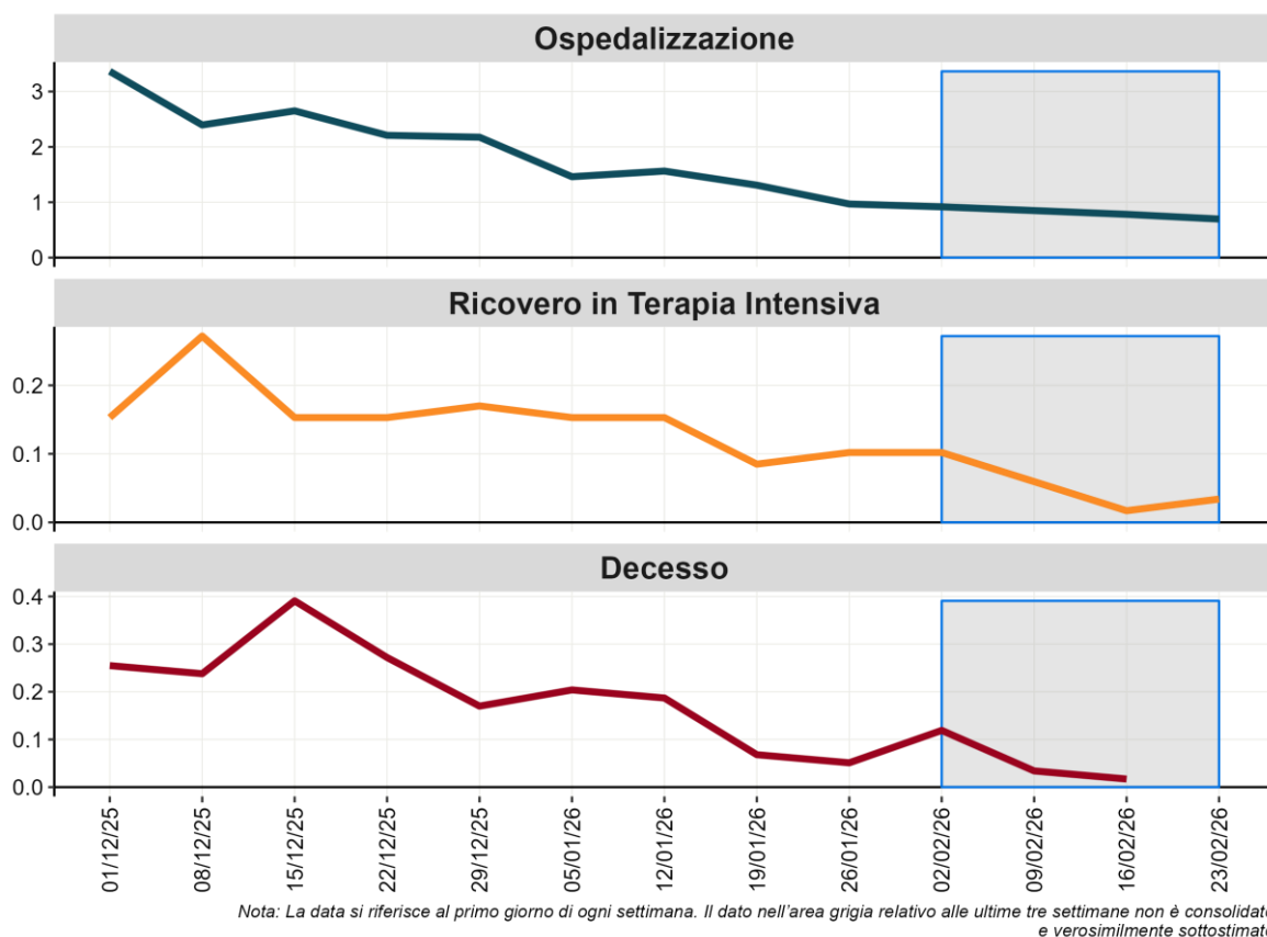
Figura 12 - Tasso settimanale di ospedalizzazione, ricovero in terapia intensiva e decesso in pazienti con diagnosi di infezione da SARS-CoV-2 (per 1.000.000 ab.), a partire dall'1 dicembre 2025
