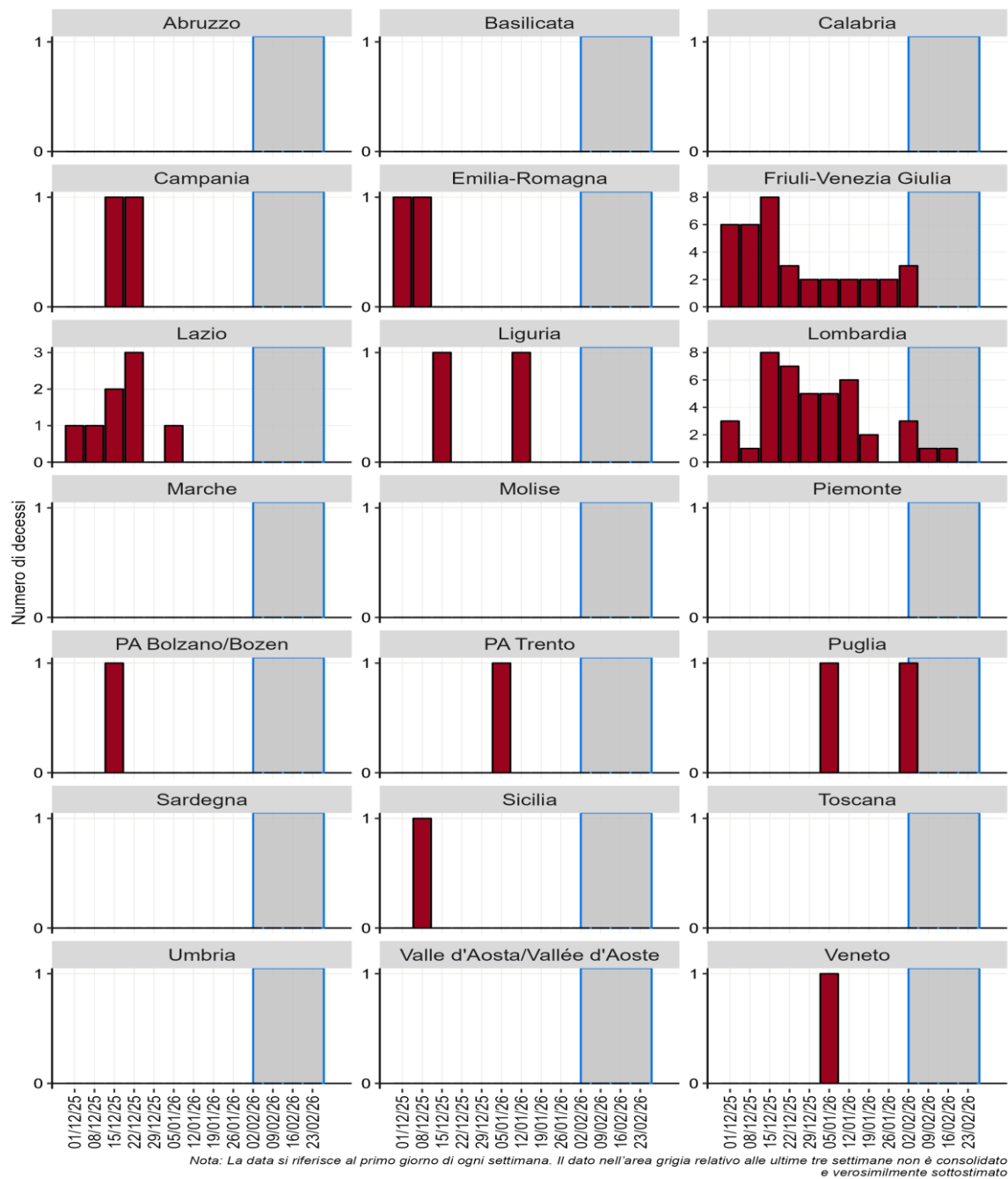
Figura 21 - Decessi settimanali per Regione/PPAA dall'1 dicembre 2025
