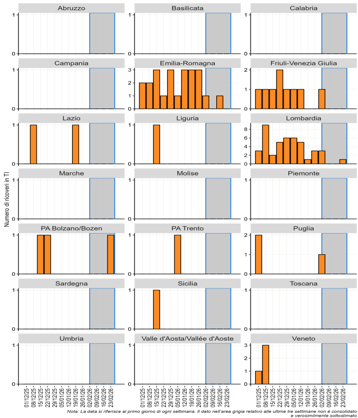
Figura 23 - Ricoveri settimanali in TI per Regione/PPAA dall'1 dicembre 2025
