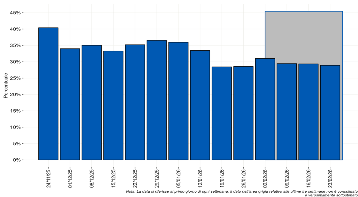
Figura 9 - Distribuzione percentuale settimanale delle diagnosi di reinfezione da SARS-CoV-2 sul totale delle diagnosi segnalate per data di prelievo/diagnosi a partire dall'1 dicembre 2025
