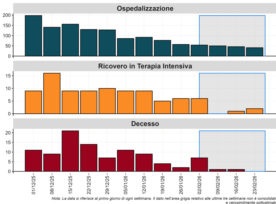
Figura 11 - Numero settimanale di ospedalizzazioni, ricoveri in terapia e decessi per settimana dell'evento a partire dall'1 dicembre 2025
