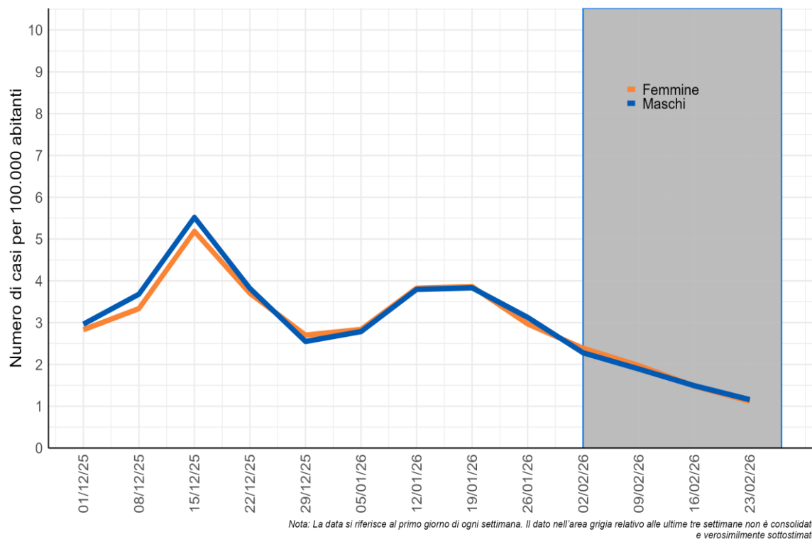
Figura 3 - Incidenza settimanale di diagnosi di infezione da SARS-CoV-2 per 100.000 abitanti per sesso a partire dall'1 dicembre 2025
